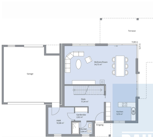
Haus Daume Grundriss
